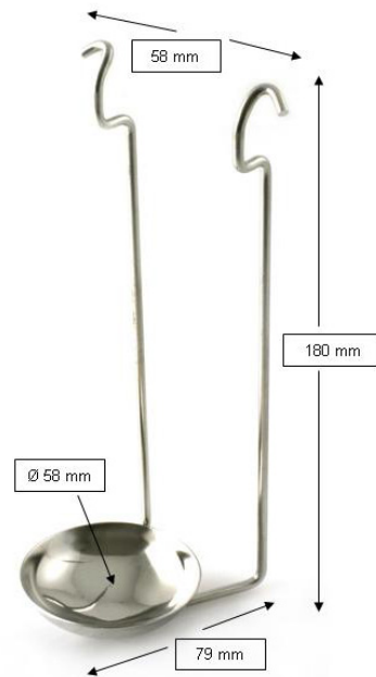
Tippa-alusta dispenser-telineelle 8155
